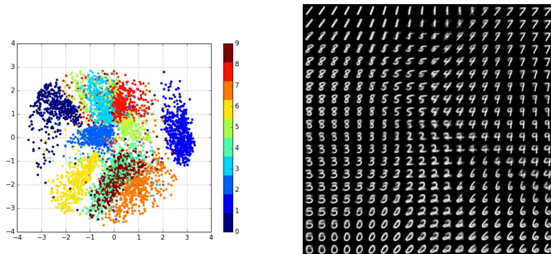
(a) 训练集上所有样本在隐空间上的投影。
