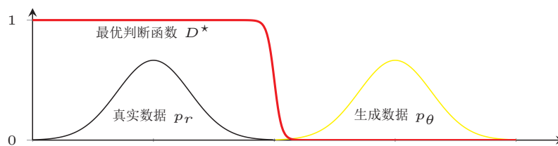
图 13.9 生成对抗网络中的梯度消失问题
