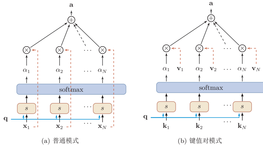
图 8.1 注意力机制
