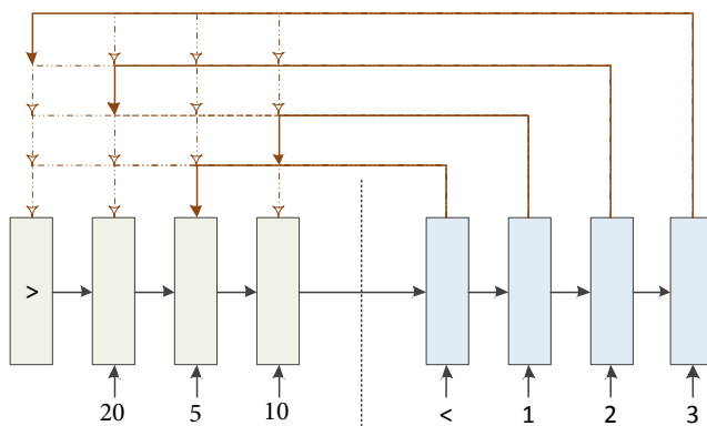
图 8.2 指针网络
