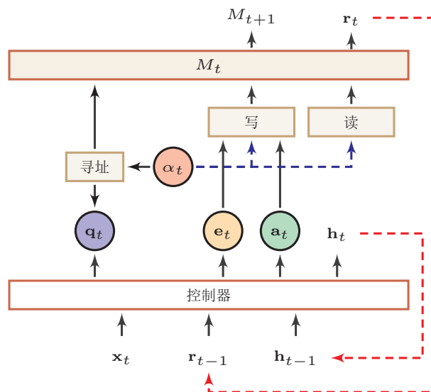
图 8.6 神经图灵机示例
