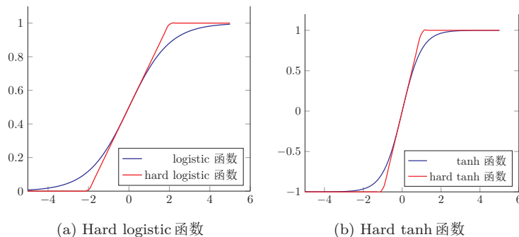
图 4.3: Hard Sigmoid 型激活函数近似
