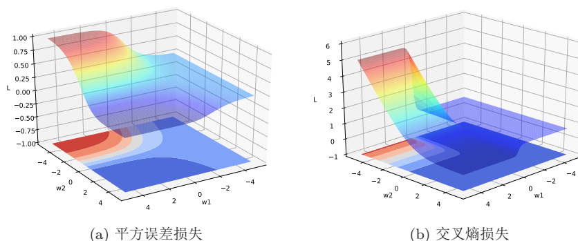
图 4.9: 损失函数与参数。1-1-1 结构神经网络为 y = \sigma(w_2\sigma(w_1x)) 。当 x = 1, y = 1 时, 其平方误差和交叉熵损失函数分别为: \mathcal{L}(w_1, w_2) = (1-y)^2 和 \mathcal{L}(w_1, w_2) = \ln y
