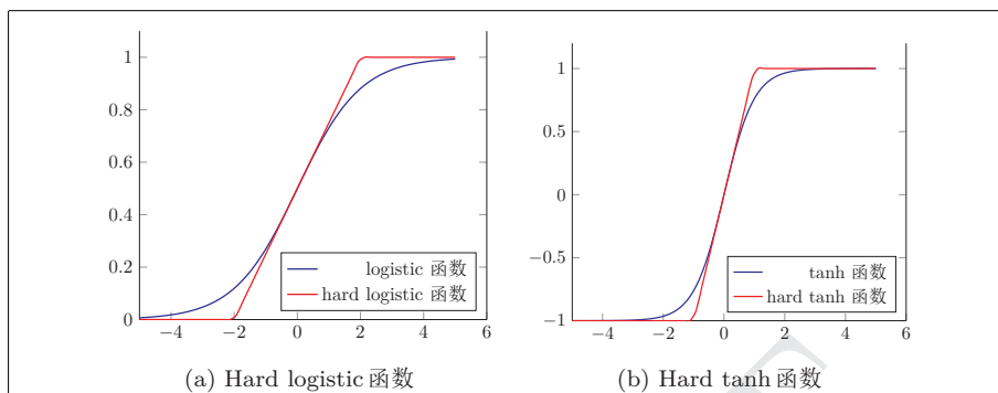
图 5.3: Sigmoid 型激活函数近似
